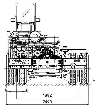
Tampak Belakang
