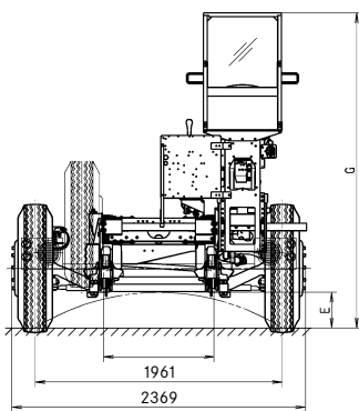
Tampak Depan
